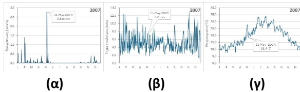
Διαγράμματα 2 (α) – (γ): Μέση τιμή της βροχόπτωσης, της ταχύτητας του ανέμου και της θερμοκρασίας σε ημερήσια βάση.
