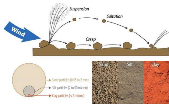
Εικόνα 3: Ο τρόπος που τα σωματίδια σκόνης κινούνται μέσα στην ατμόσφαιρα (Darvishi Boloorani et al., 2023)
