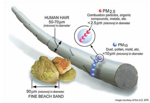
Εικόνα 2: Το μέγεθος των αιωρούμενων σωματιδίων σε σύγκριση με την ανθρώπινη τρίχα (EPA, 2023).
